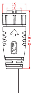
PIN 1 : BRUN (DC +) PIN 2 : BLEU (DC -)
