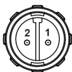
PIN 1 : BRUN (DC +) PIN 2 : BLEU (DC -)
